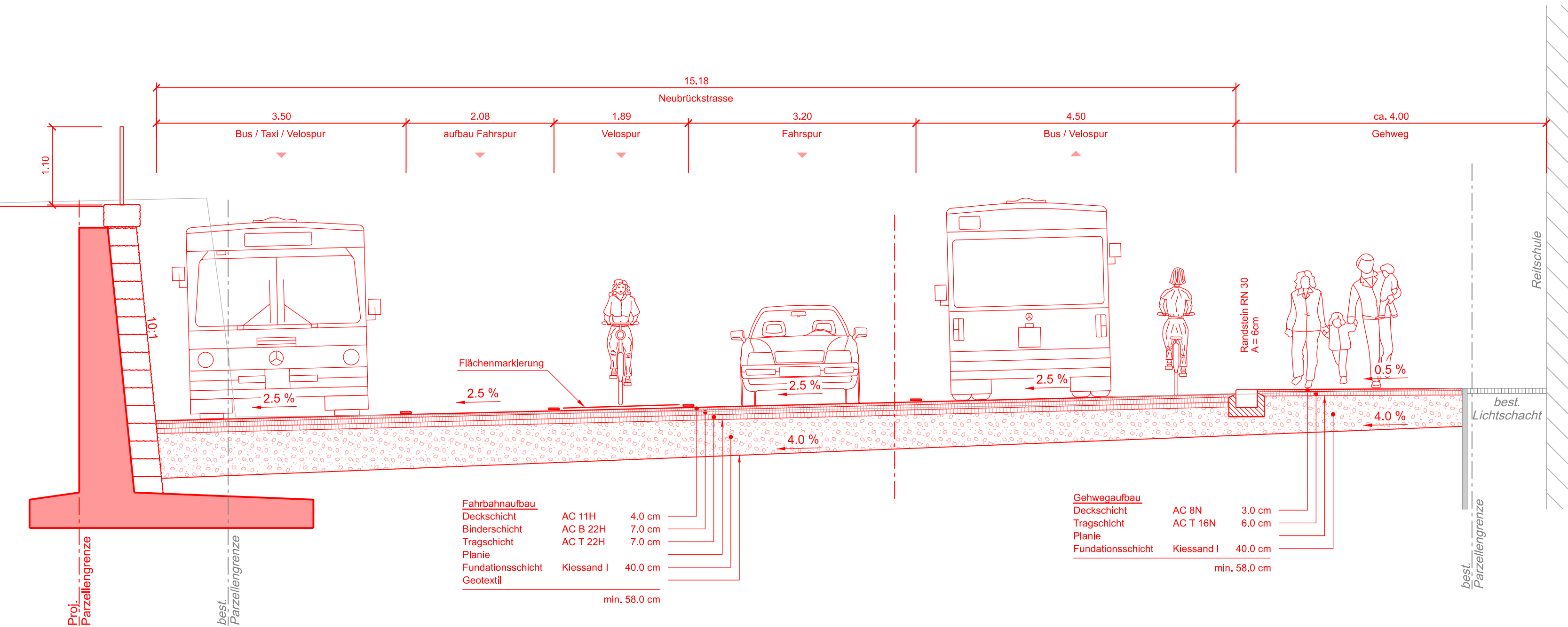
Normalprofil Neubrückstrasse 1:50
