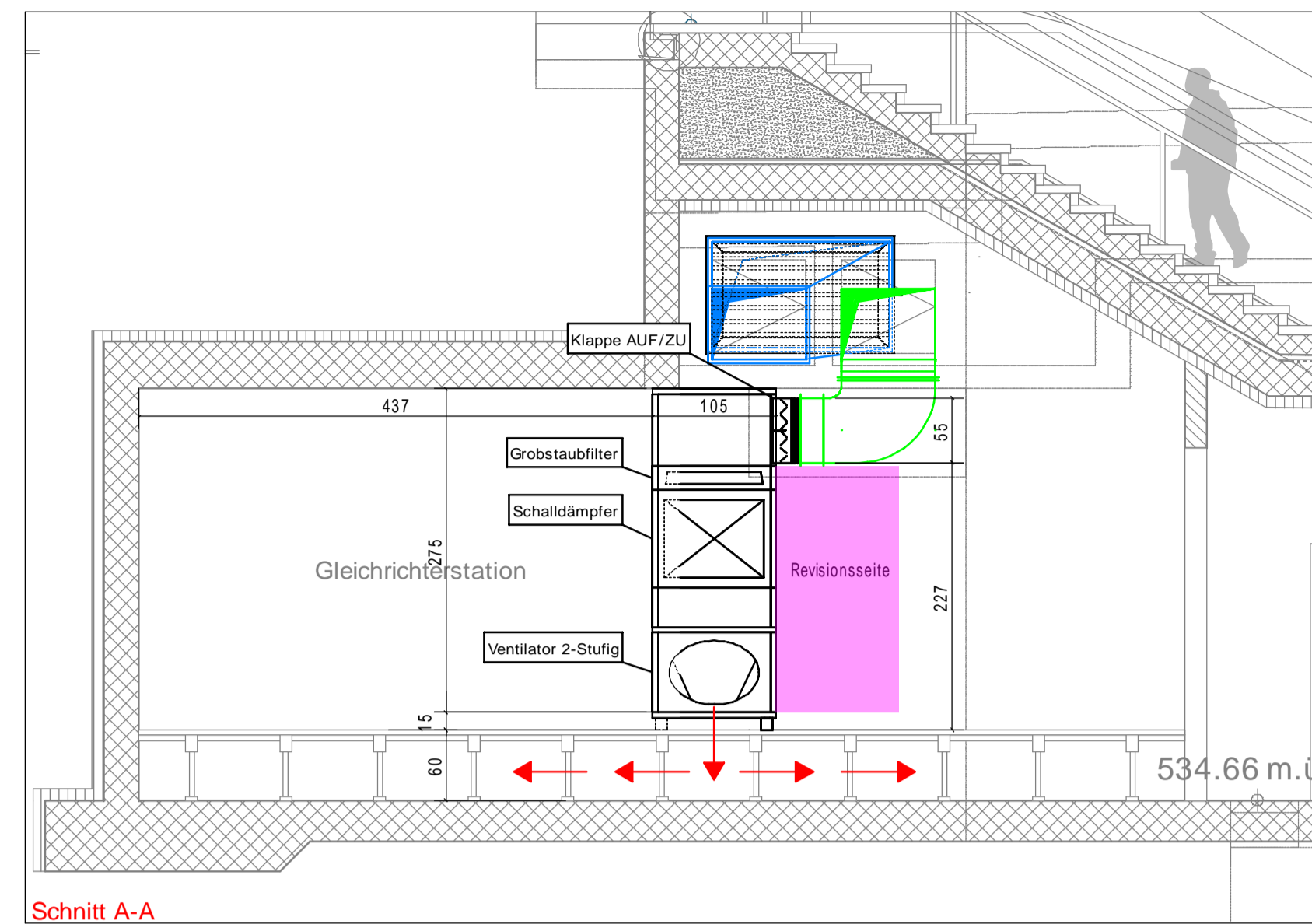
Schnitt A-A
